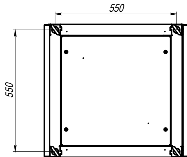
Транспортировочные болты
