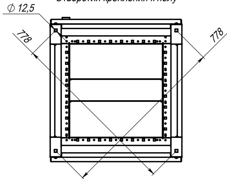
Отверстия крепления к полу
