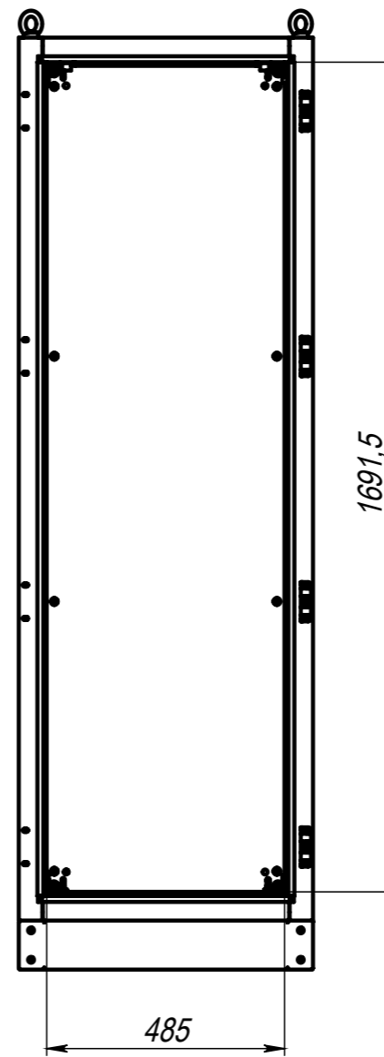
Панель монтажная
